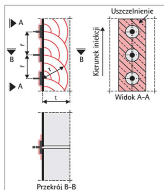
Układ iniektorów przyklejanych i kierunek iniekcji
