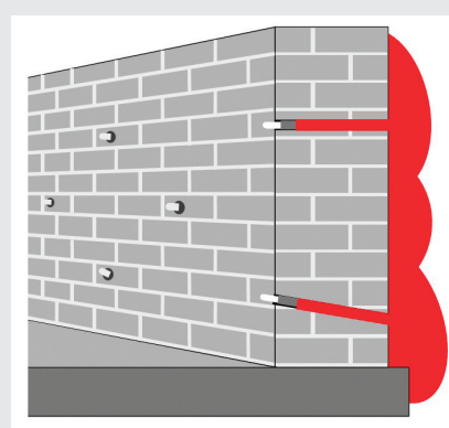
Schemat iniekcji kurtynowej
