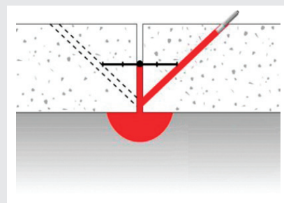
Uszczelnienie dylatacji
