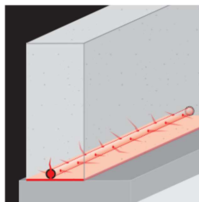
Uszczelnianie przerw roboczych za pomocą węża iniekcyjnego
