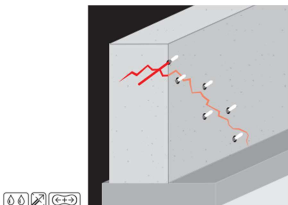
Naprawa rys w betonie
